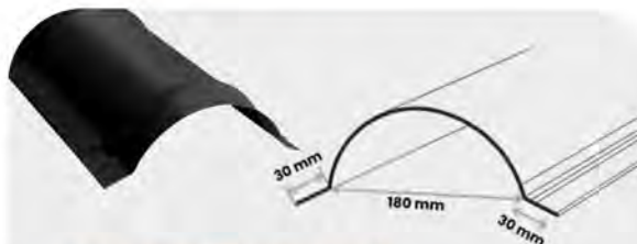
COAMĂ ROTUNDĂ
